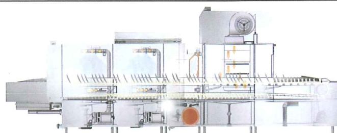
入口段 洗滌1 洗滌2 沖洗段 烘乾段 出口段
